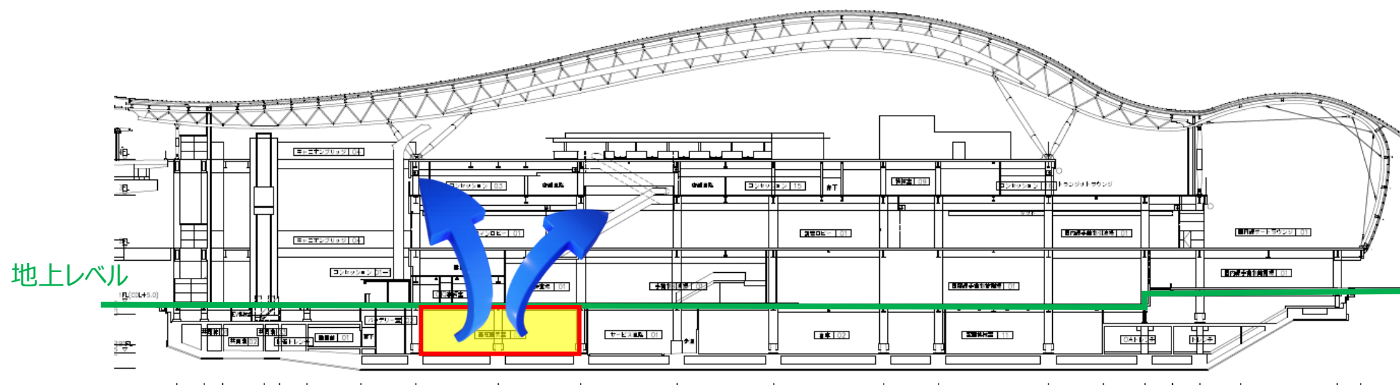
第1ターミナルビル本館 断面図
